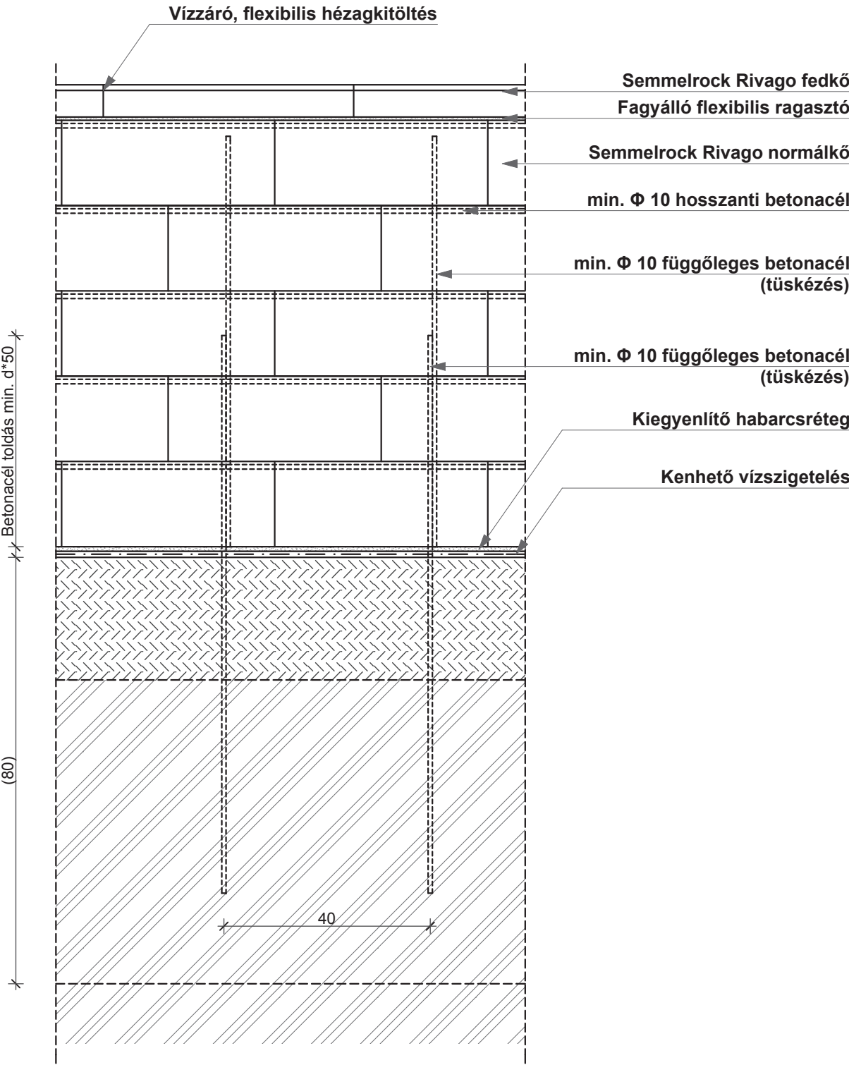
ELŐLNÉZET M=1:20
