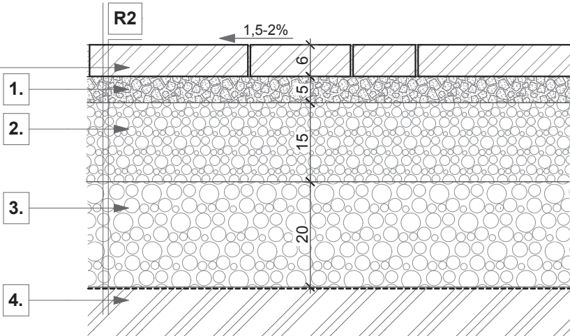
Térkő burkolat 6 cm vtg. gépjármű forgalom számára
