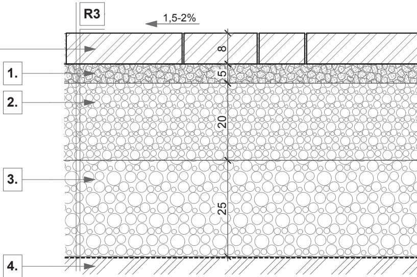
Térkő burkolat 8 cm vtg. teher fogalom számára
