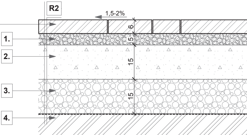
Térkő burkolat 6 cm vtg. gépjármű és gyalogos forgalom számára
