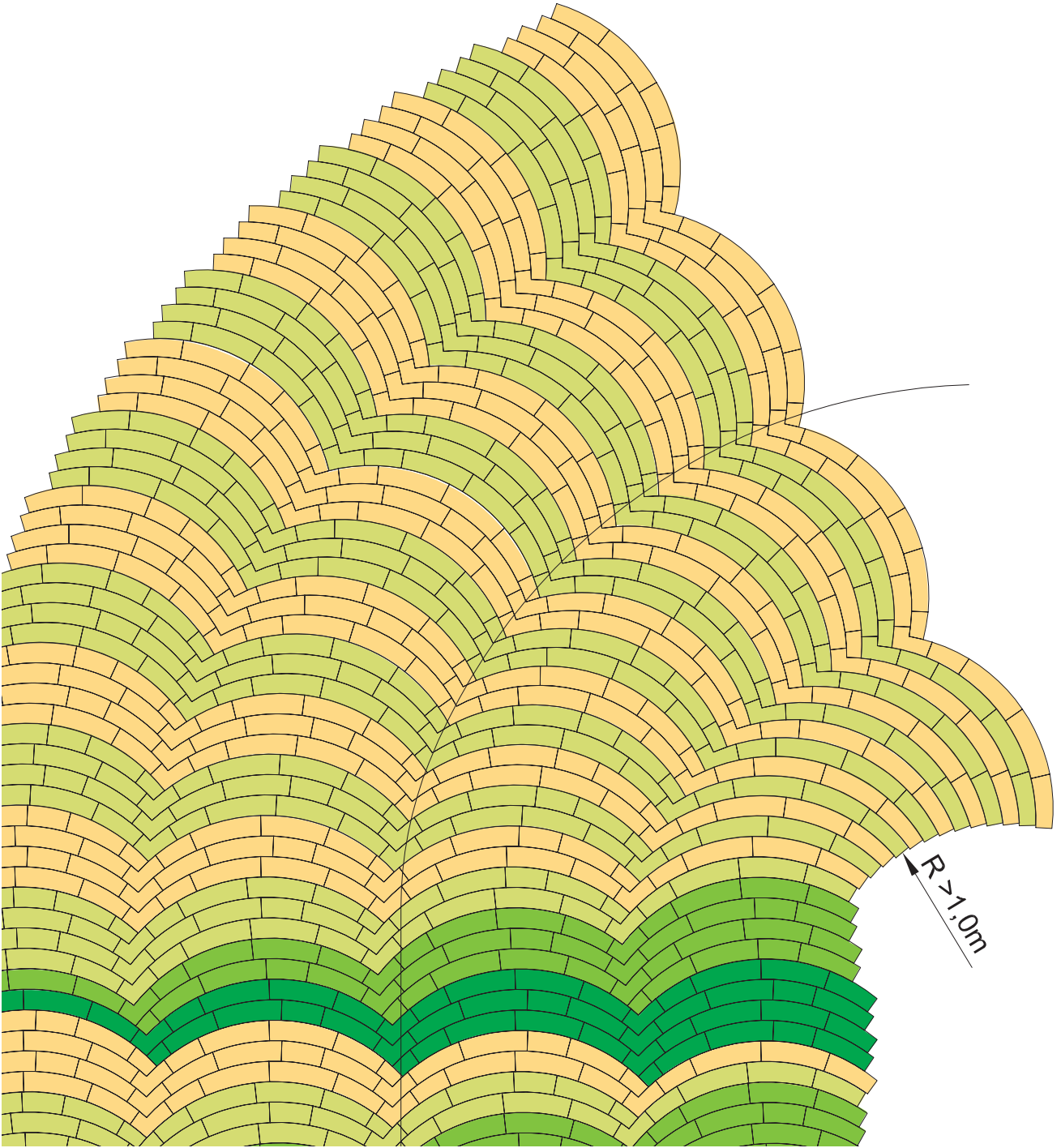
24. ábra: A fordulás minimum 1 méter belső sugarú körnél valósítható meg. A balra, illetve jobbra fordulásnál értelemszerűen csak balos vagy jobbos írendszereket használunk.
