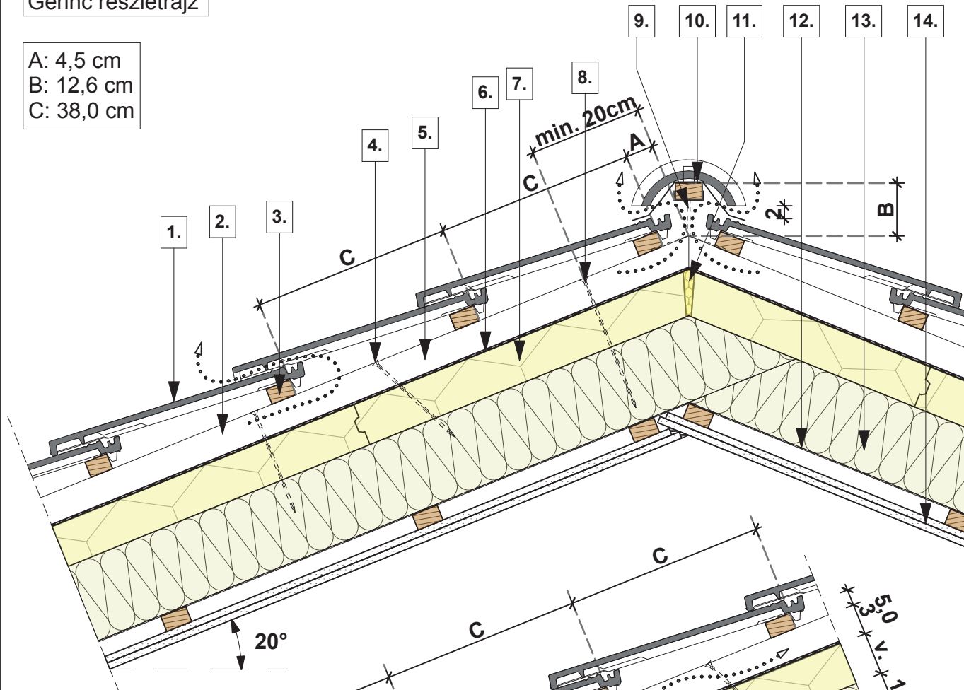
Eresz részletrajz
