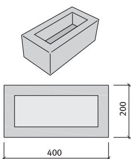
normálkő
