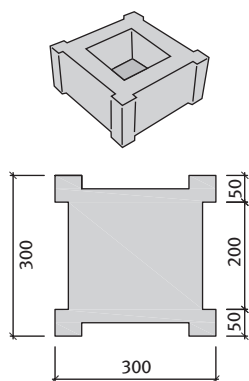
oszlopkő
