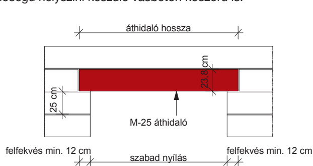
Alkalmazás egyszerű áthidalóként
